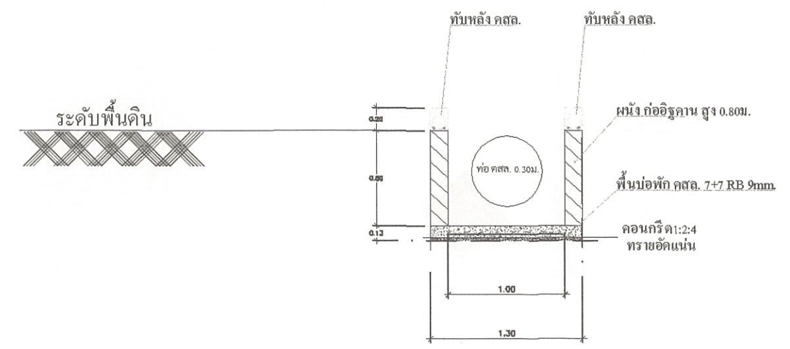
รูปตัดบ่อพักน้ำเสีย SCALE 1:100
