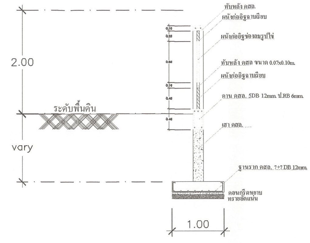
แบบขยายรั้ว C SCALE 1:100
